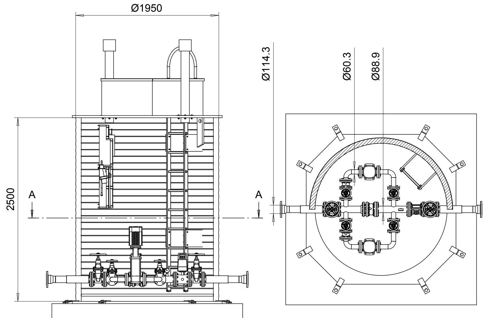
A-A 1:30
